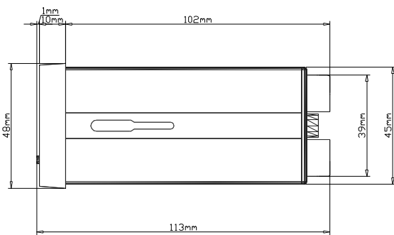
Fig. 4 – Vista lateral
