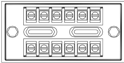
Fig. 2 – Vista posterior
