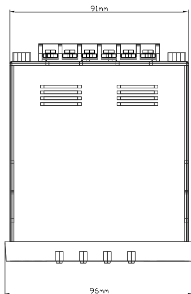
Fig. 5 – Vista superior
